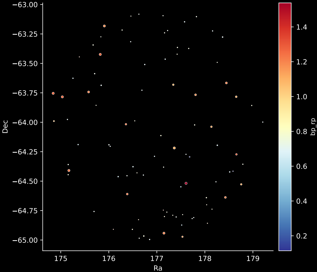
GALAH DR4 Field: [7137] Stars: 92
