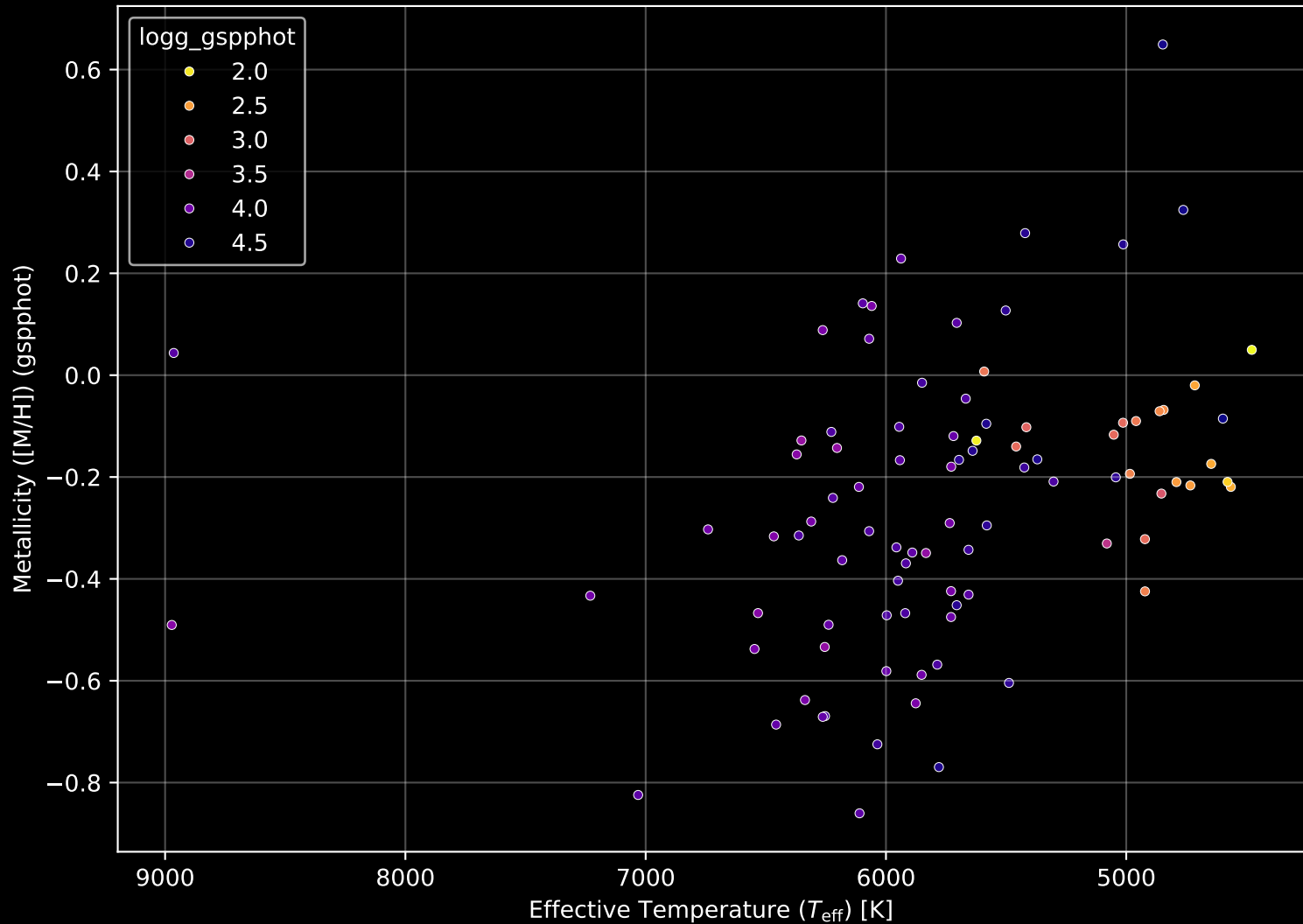
GALAH DR4 Field: [7137] Stellar Population Parameters (n= 92)
