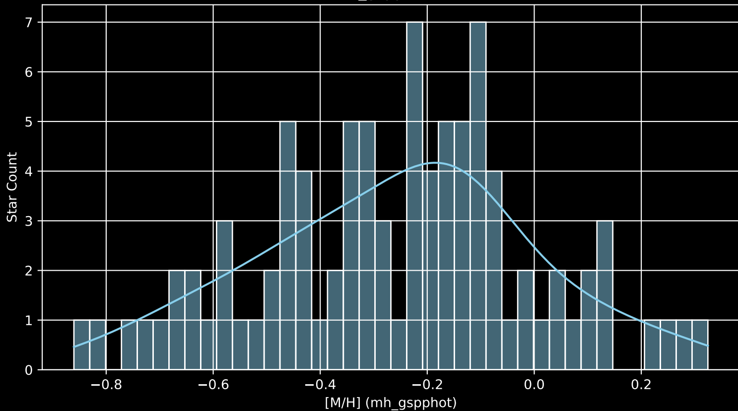
GALAH DR4 Field: [7137] [M/H] (mh_gspphot) (n= 91)
